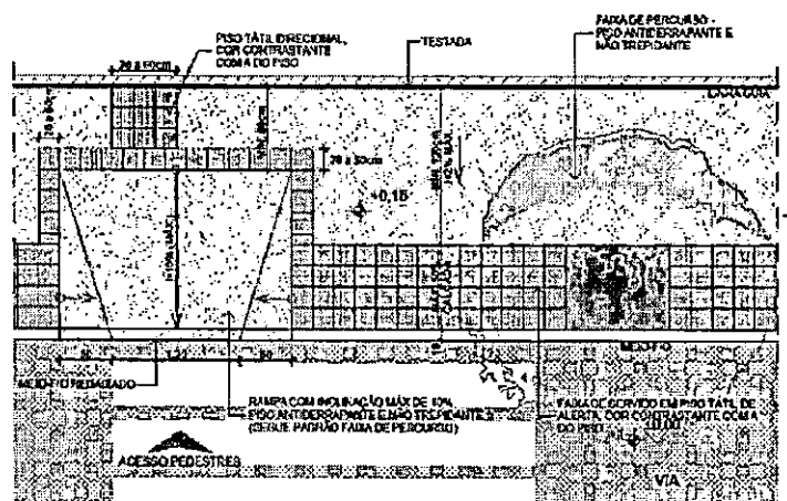
Calçadas com 3ª faixa L > 230\text{cm}
