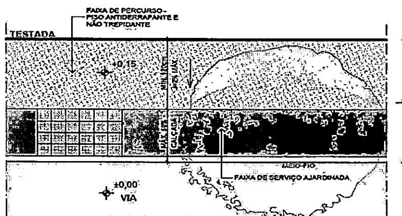
Calçadas sem 3ª faixa
