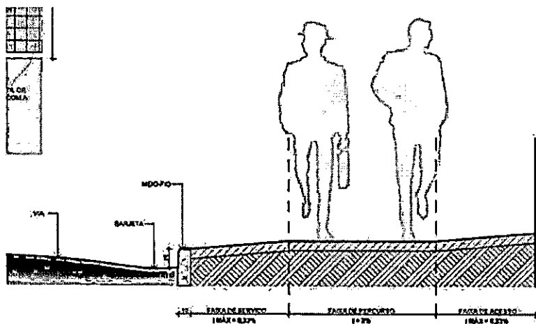
Corte Transversal da calçada com 3ª Faixa – Exemplo
